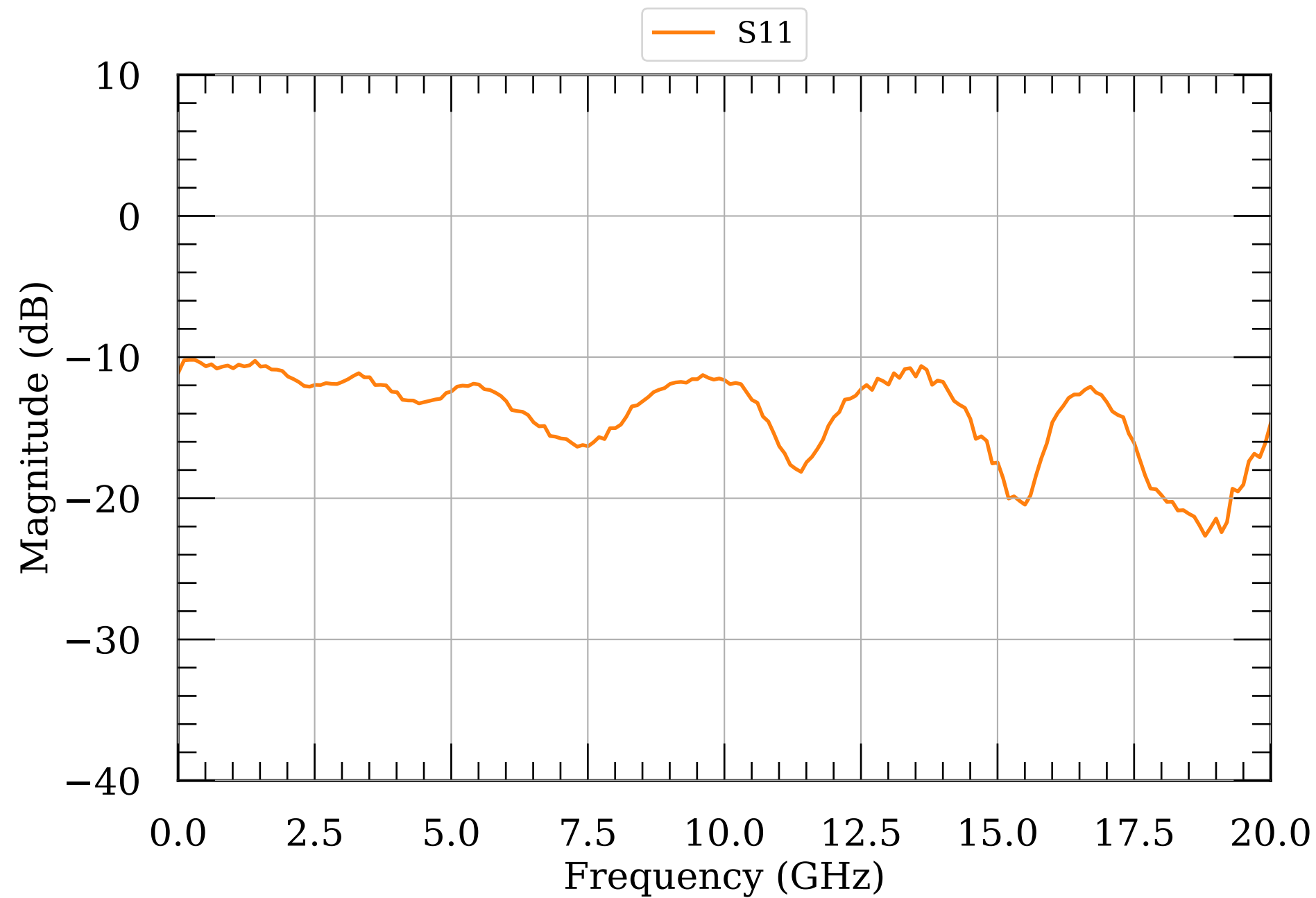
LNA S-params module062
